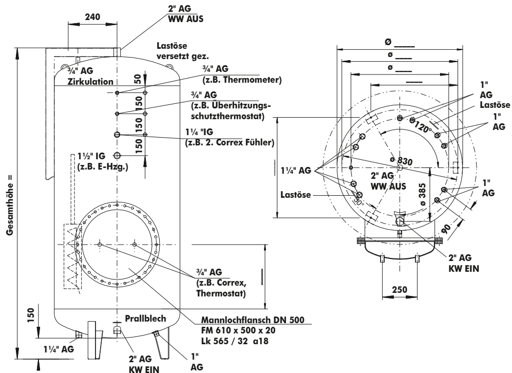
Vorderansicht
