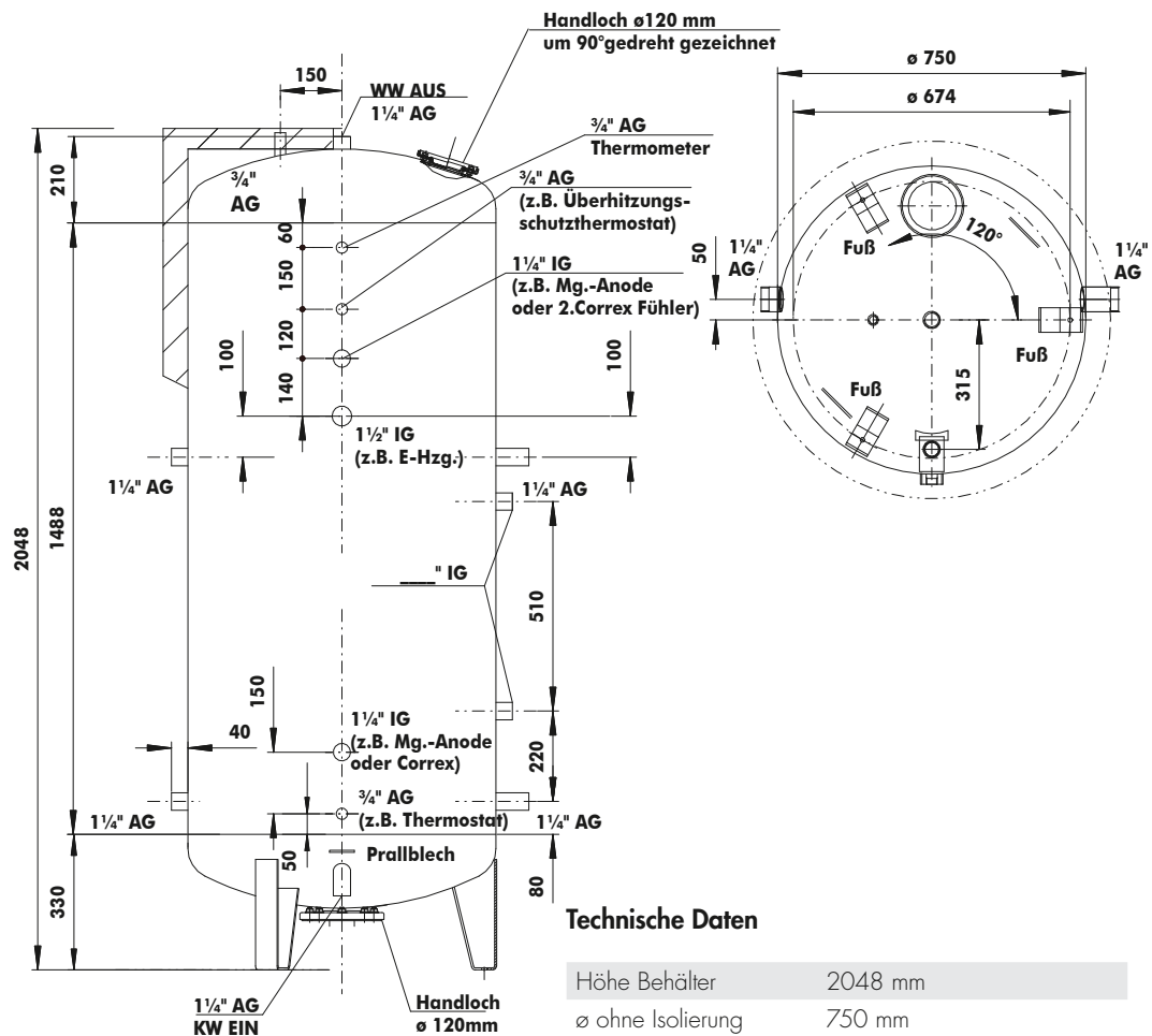
Vorderansicht
